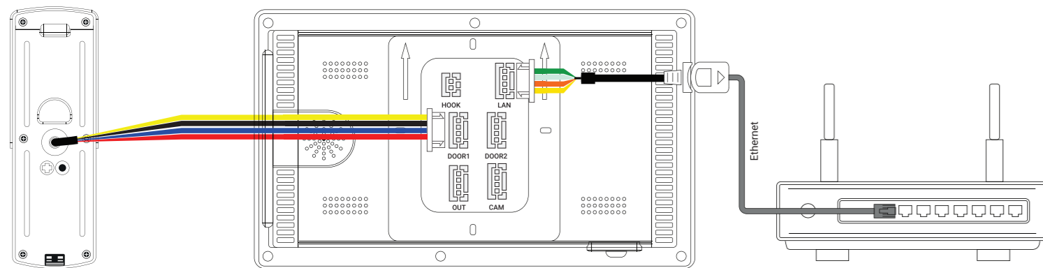
Схема підключення однієї панелі і дротового підключення до інтернету. Схеми підключення додаткових пристроїв дивіться у докладній інструкції по експлуатації.
