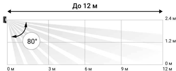
Вертикальный угол обзора датчика
